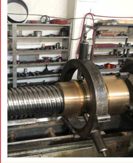
Q310 DÖRT AĞIZLI VİDA VE SOMUNU
